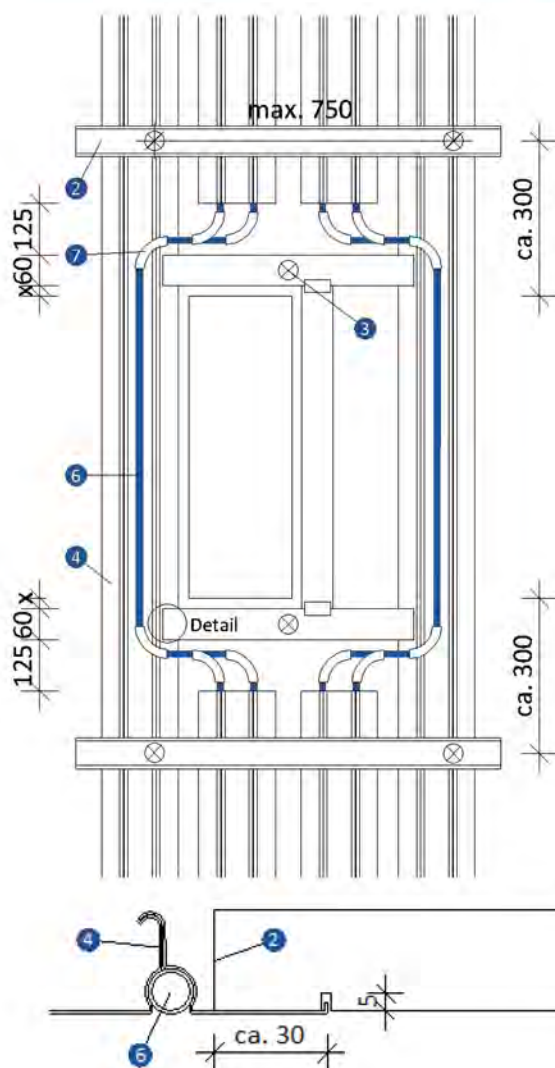
DA6.1 – REGELDETAIL FÜR LAMPENAUSSWECHSLUNG MIT UMLENKVERROHRUNG
