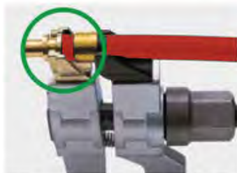
Richtig ausgerichtet in MSZ Schiebebacke F.
